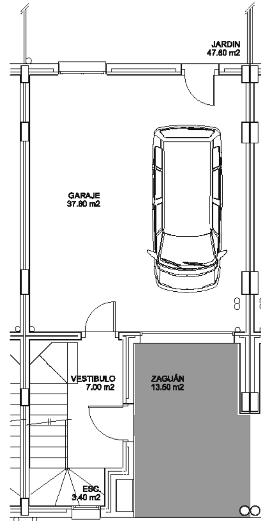
planta baja
