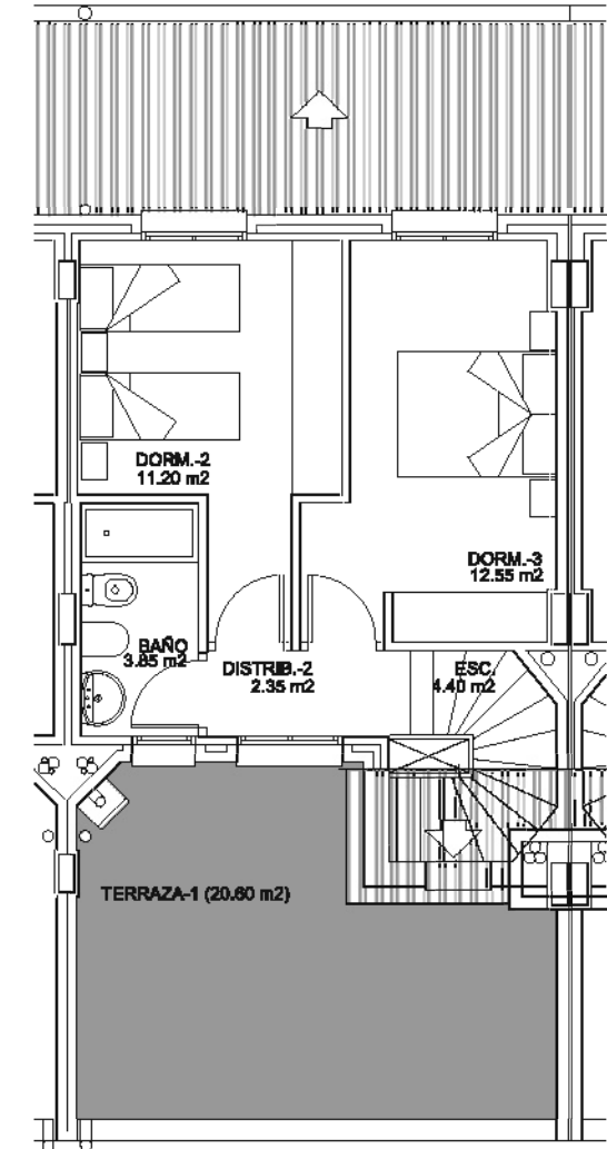
planta segunda
