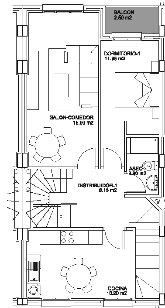
planta primera
