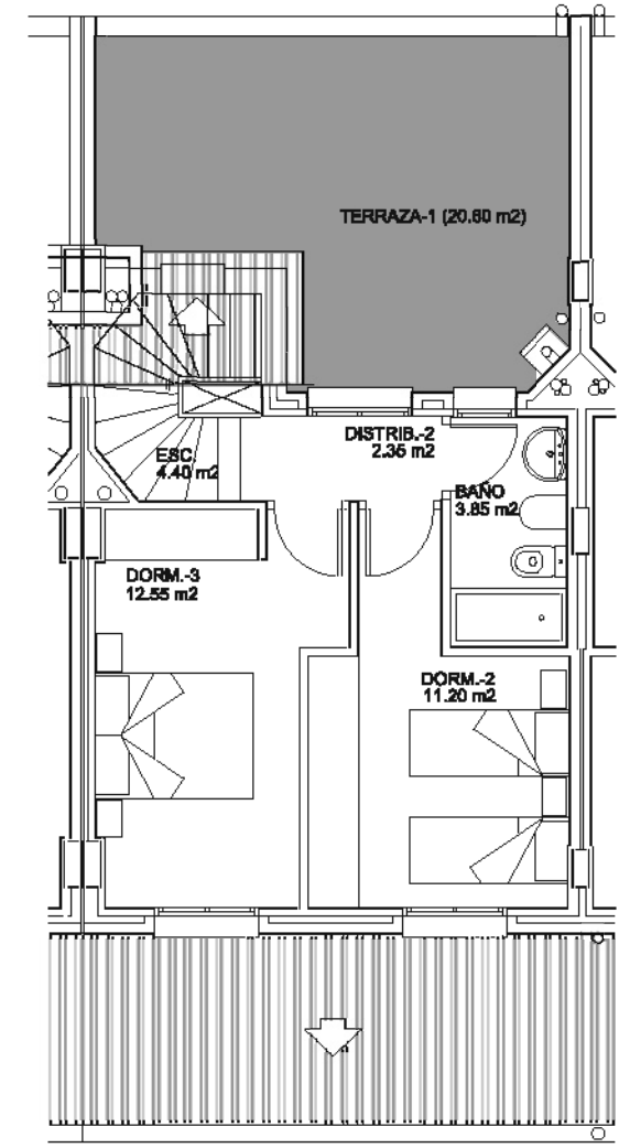
planta segunda
