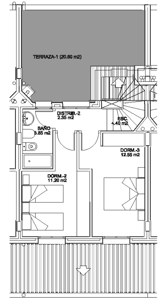
planta segunda
