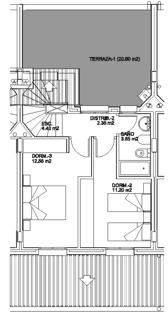
planta segunda
